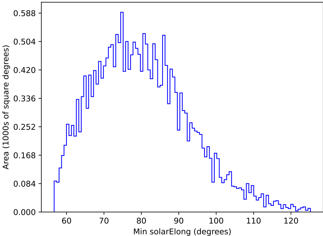
extra_ss_neo3_v3.4_10yrs All sky u band: Min solarElong
