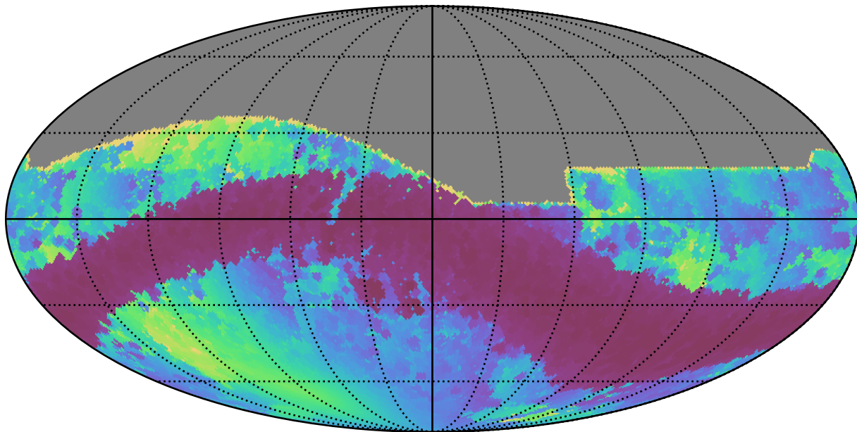
extra_ss_neo3_v3.4_10yrs All sky r band: Min solarElong
