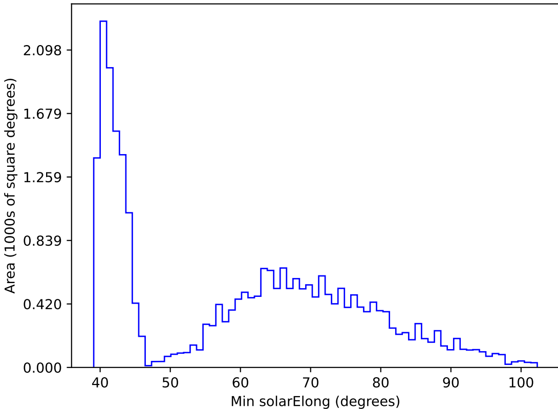
extra_ss_neo3_v3.4_10yrs All sky r band: Min solarElong
