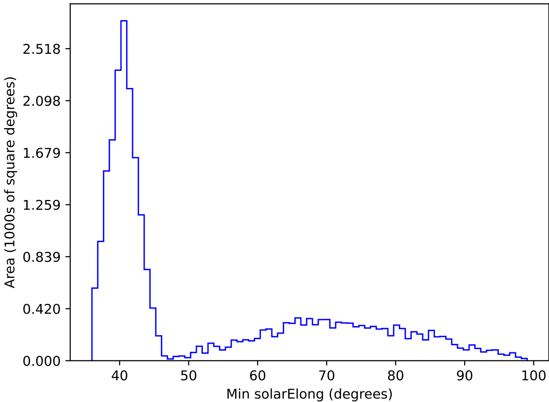
extra_ss_neo3_v3.4_10yrs All sky i band: Min solarElong
