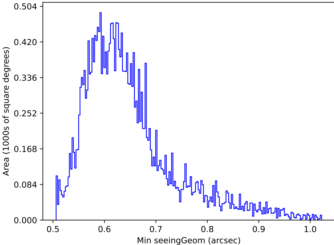
extra_ss_neo3_v3.4_10yrs Yr 1 z band: Min seeingGeom
