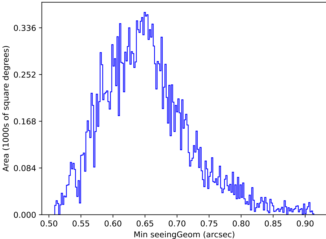
extra_ss_neo3_v3.4_10yrs Yr 1 y band: Min seeingGeom
