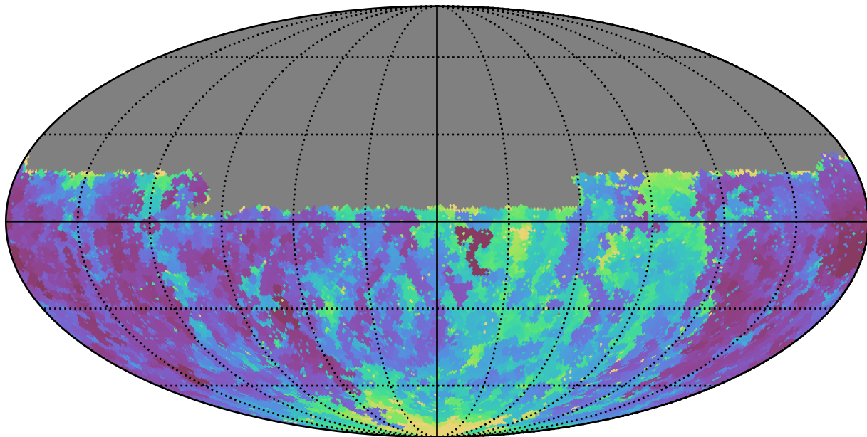
extra_ss_neo3_v3.4_10yrs Yr 1 u band: Min seeingGeom
