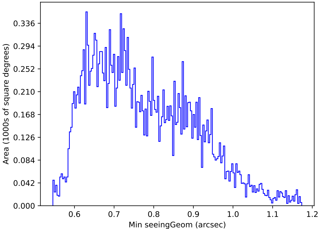
extra_ss_neo3_v3.4_10yrs Yr 1 u band: Min seeingGeom
