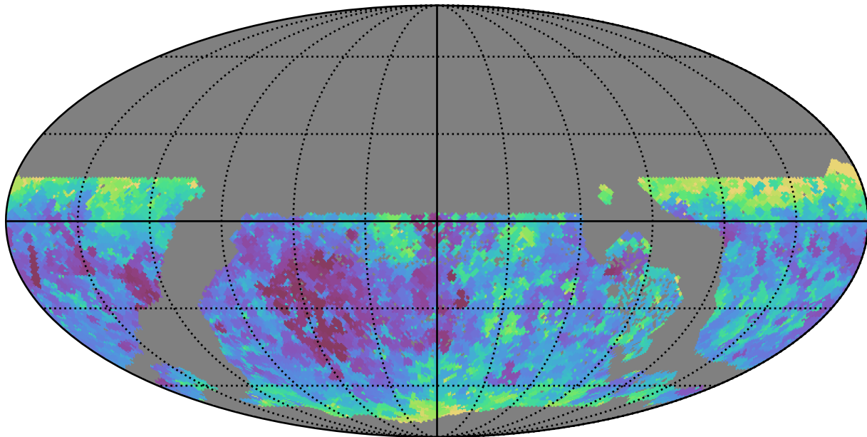
extra_ss_neo3_v3.4_10yrs WFD y band: Min seeingEff
