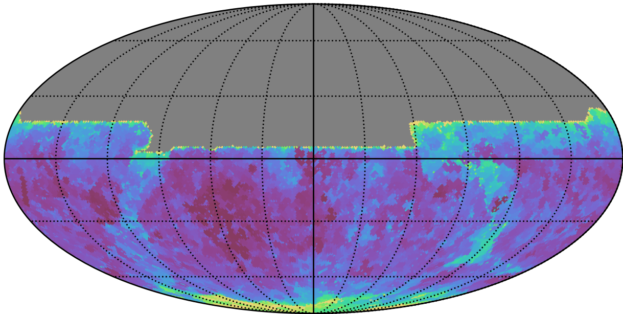
extra_ss_neo3_v3.4_10yrs All sky y band: Min seeingEff
