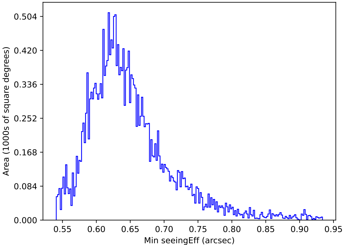
extra_ss_neo3_v3.4_10yrs All sky y band: Min seeingEff
