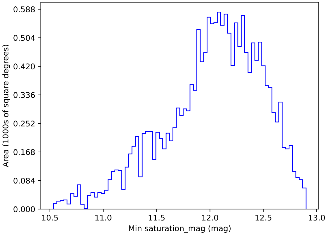
extra_ss_neo3_v3.4_10yrs WFD z band: Min saturation_mag
