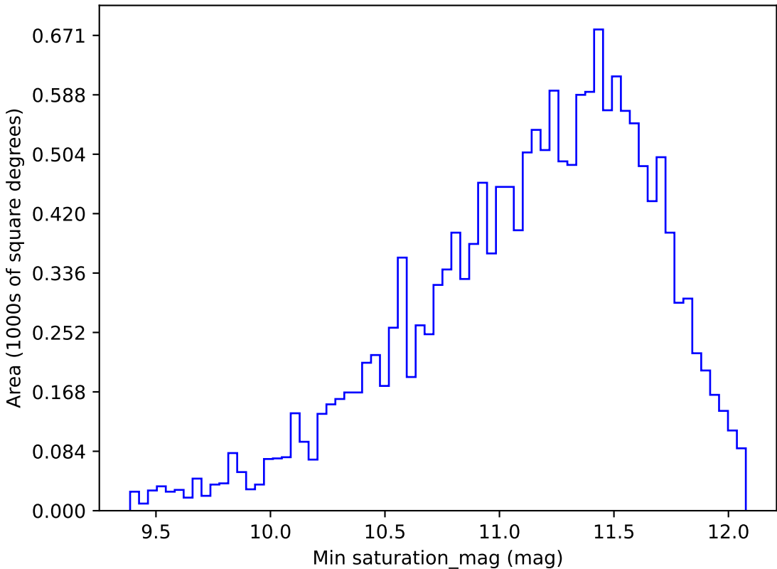
extra_ss_neo3_v3.4_10yrs WFD y band: Min saturation_mag
