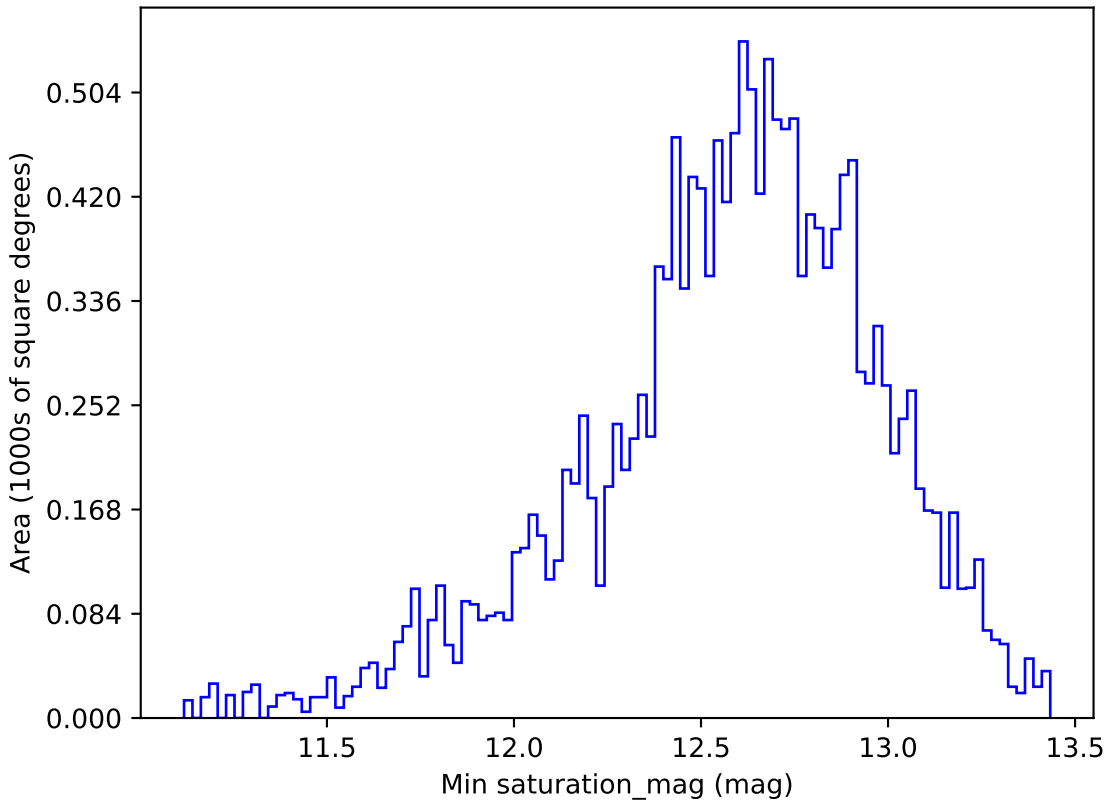
extra_ss_neo3_v3.4_10yrs WFD r band: Min saturation_mag
