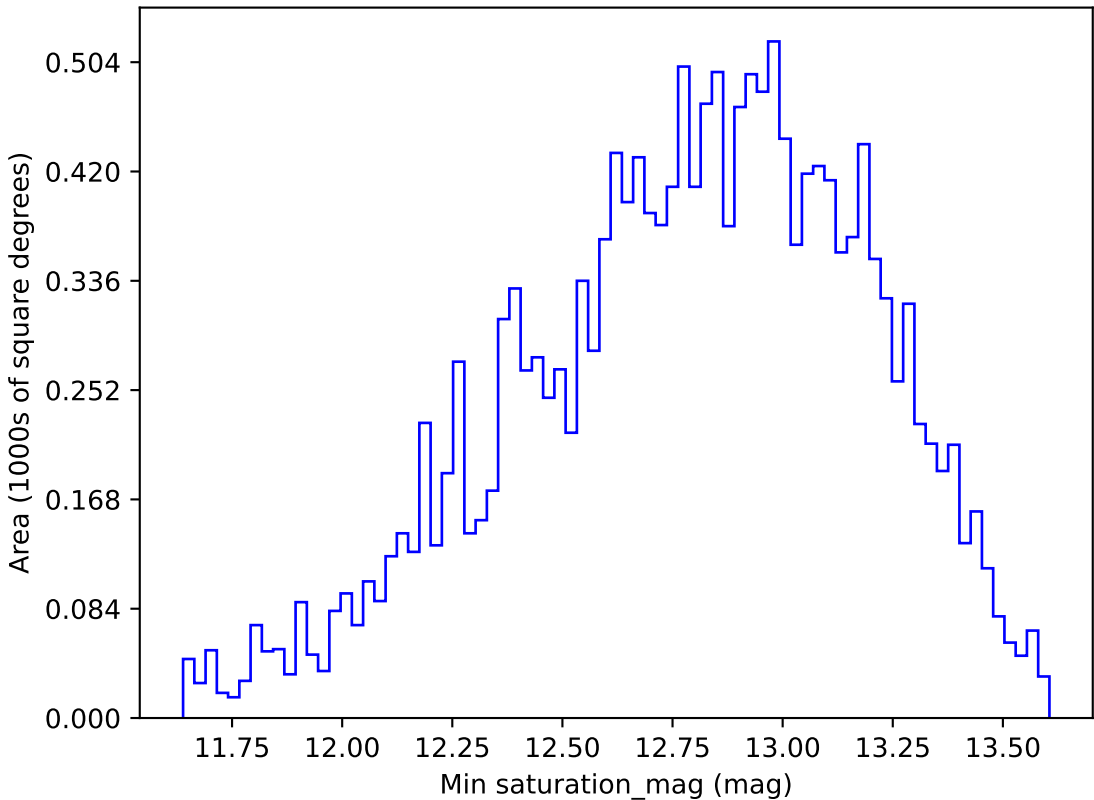
extra_ss_neo3_v3.4_10yrs WFD g band: Min saturation_mag
