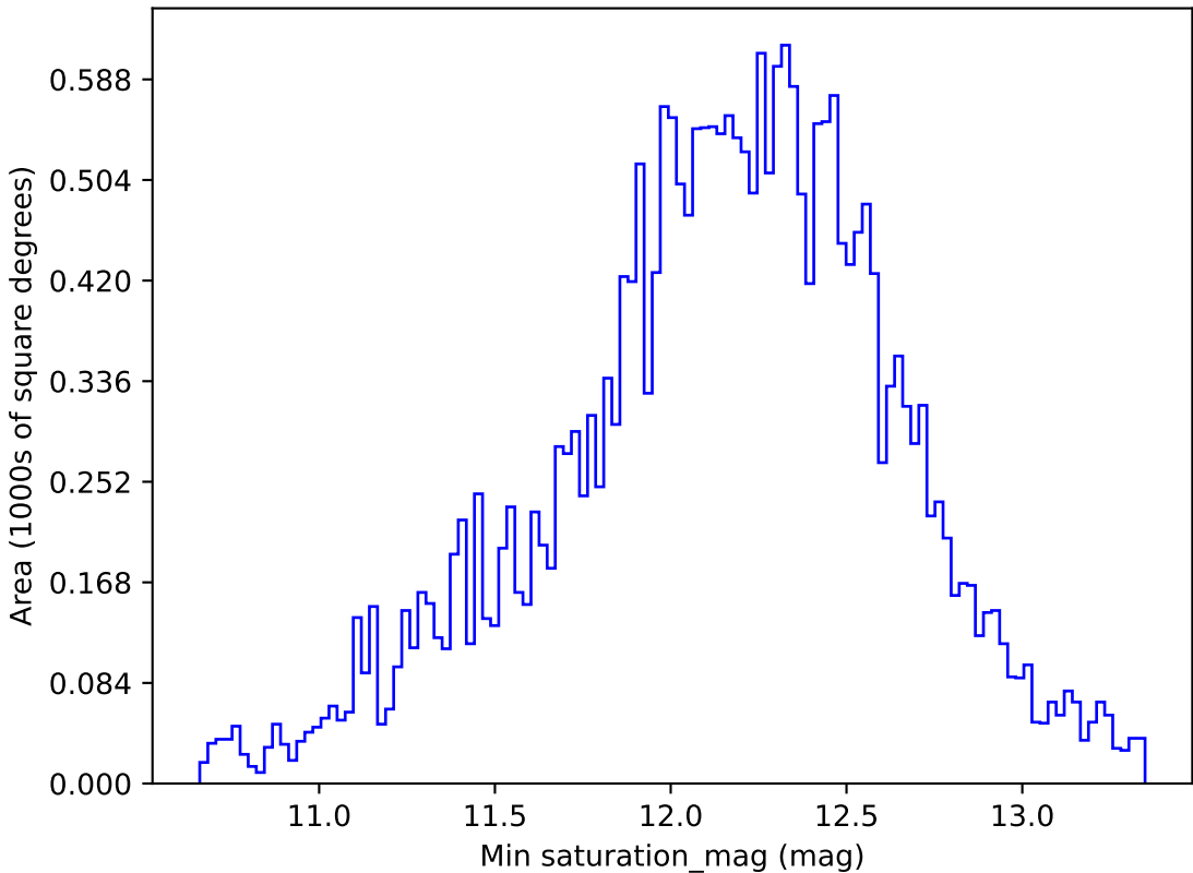
extra_ss_neo3_v3.4_10yrs All sky z band: Min saturation_mag
