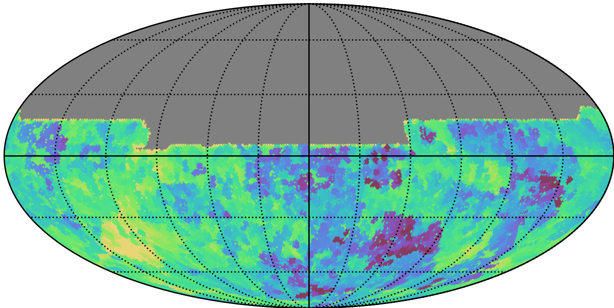
extra_ss_neo3_v3.4_10yrs All sky y band: Min saturation_mag
