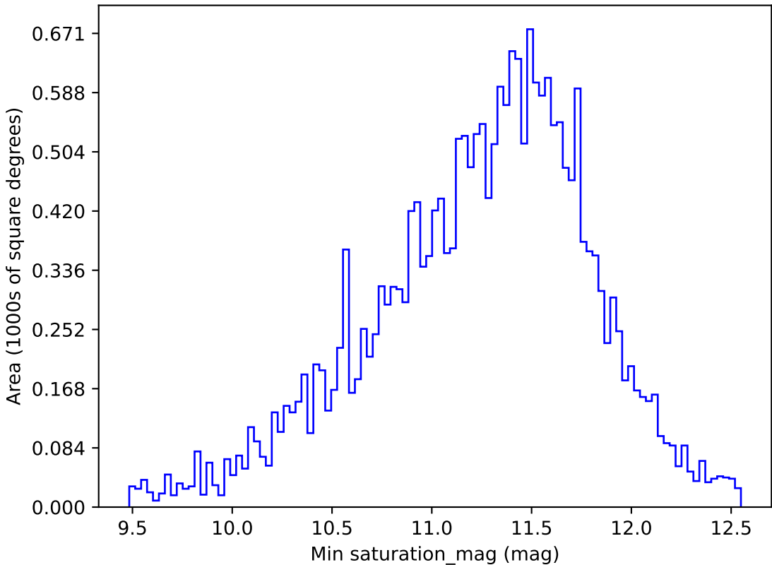
extra_ss_neo3_v3.4_10yrs All sky y band: Min saturation_mag
