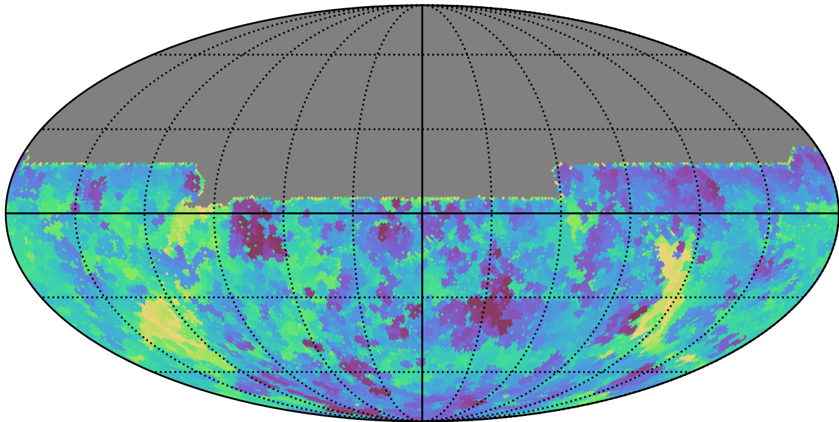
extra_ss_neo3_v3.4_10yrs All sky u band: Min saturation_mag
