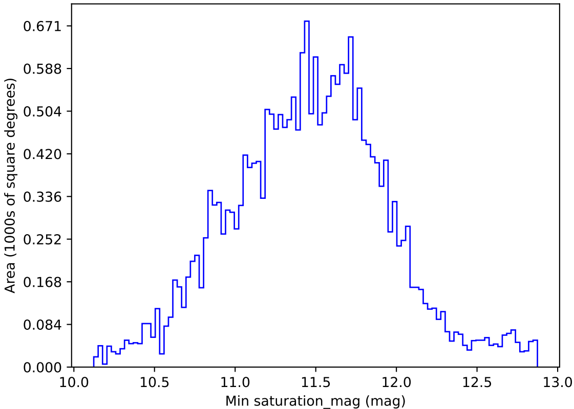
extra_ss_neo3_v3.4_10yrs All sky u band: Min saturation_mag
