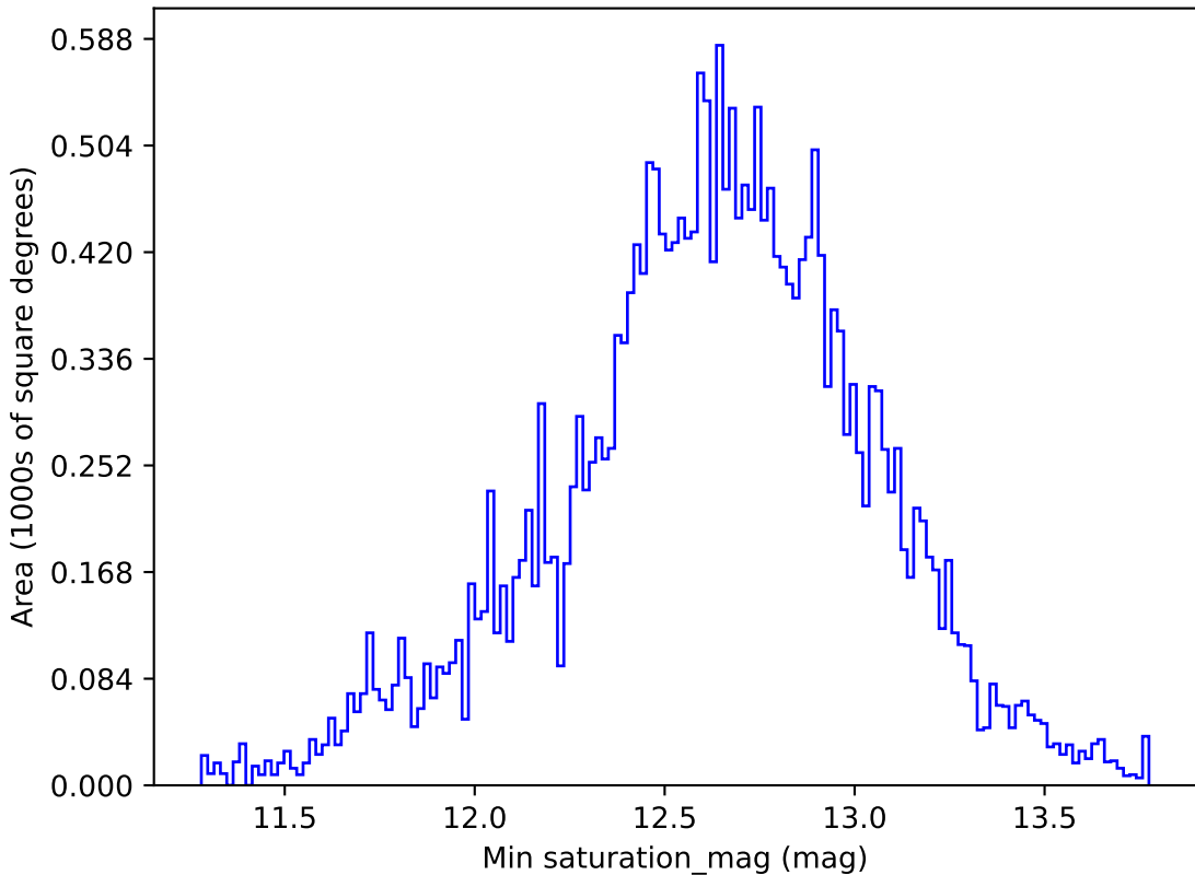
extra_ss_neo3_v3.4_10yrs All sky r band: Min saturation_mag
