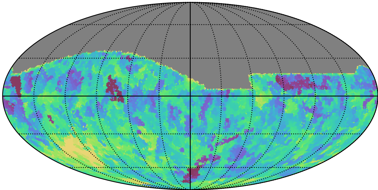
extra_ss_neo3_v3.4_10yrs All sky i band: Min saturation_mag
