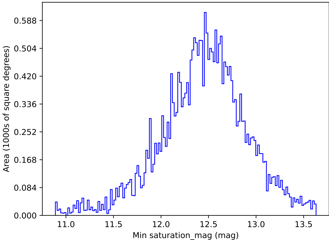
extra_ss_neo3_v3.4_10yrs All sky i band: Min saturation_mag
