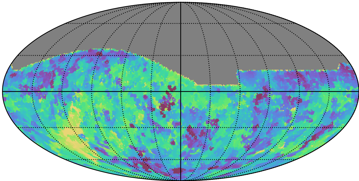
extra_ss_neo3_v3.4_10yrs All sky g band: Min saturation_mag
