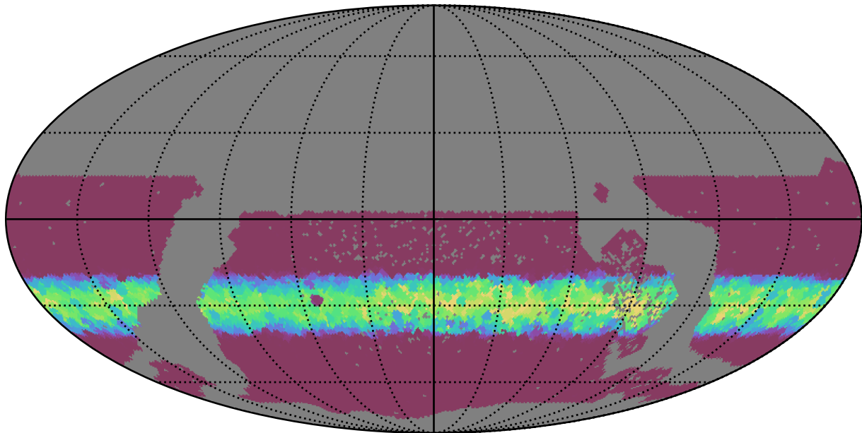
extra_ss_neo3_v3.4_10yrs WFD z band: Min normairmass
