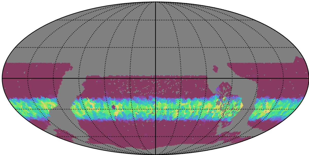
extra_ss_neo3_v3.4_10yrs WFD u band: Min normairmass
