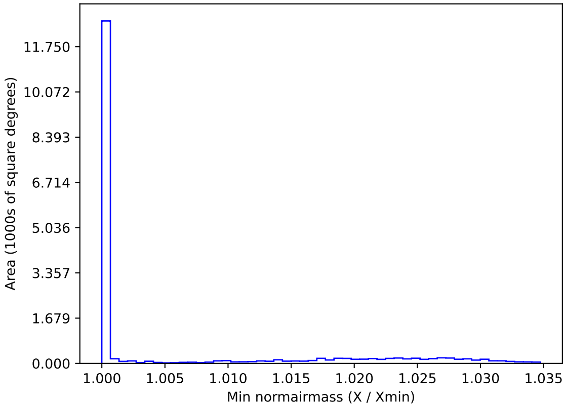
extra_ss_neo3_v3.4_10yrs WFD r band: Min normairmass
