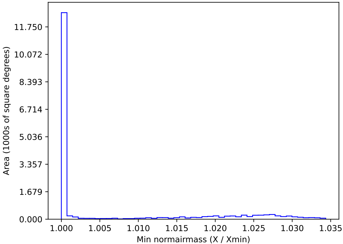
extra_ss_neo3_v3.4_10yrs WFD i band: Min normairmass
