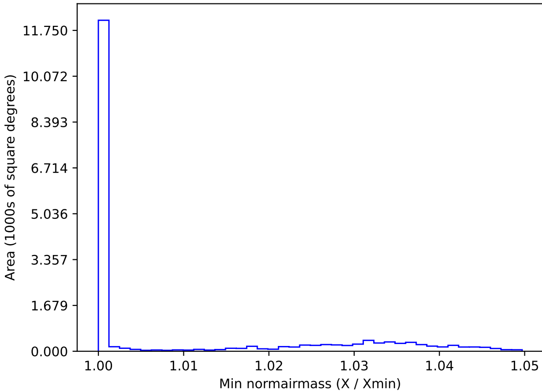
extra_ss_neo3_v3.4_10yrs WFD g band: Min normairmass
