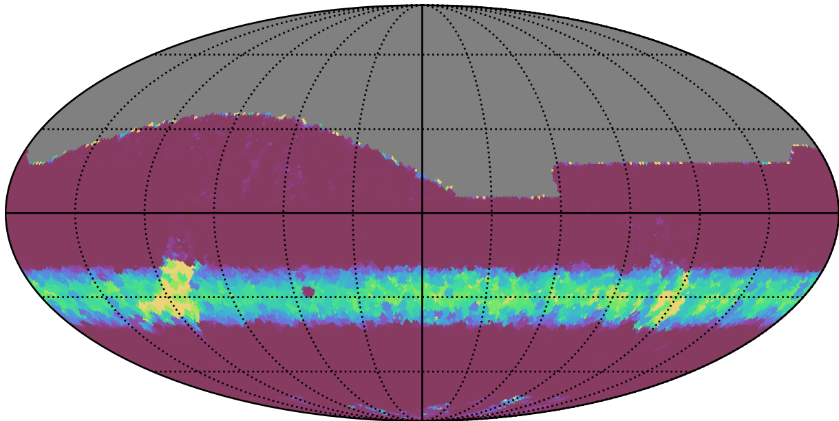
extra_ss_neo3_v3.4_10yrs All sky z band: Min normairmass
