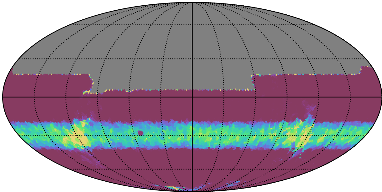
extra_ss_neo3_v3.4_10yrs All sky y band: Min normairmass
