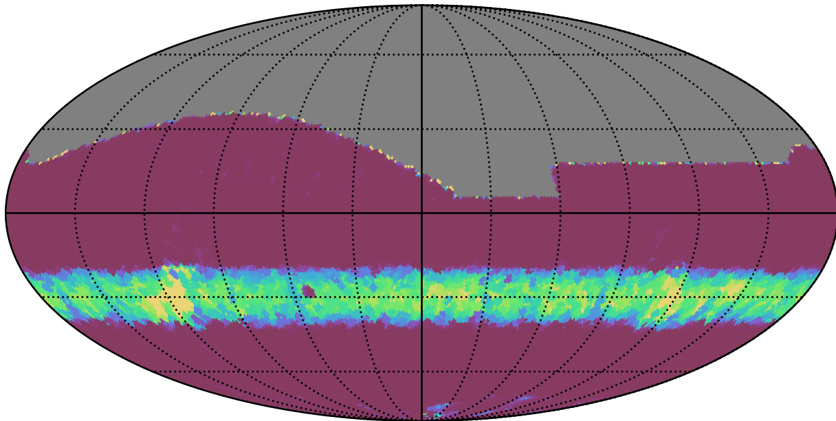
extra_ss_neo3_v3.4_10yrs All sky i band: Min normairmass
