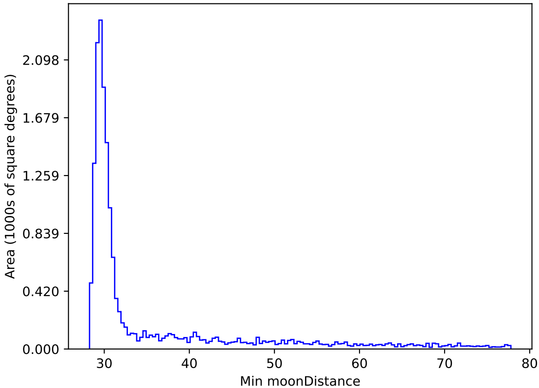
extra_ss_neo3_v3.4_10yrs WFD z band: Min moonDistance
