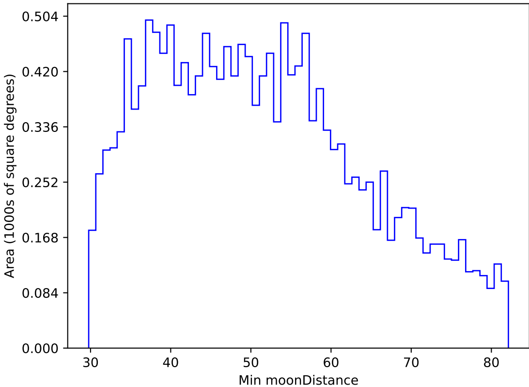
extra_ss_neo3_v3.4_10yrs WFD u band: Min moonDistance
