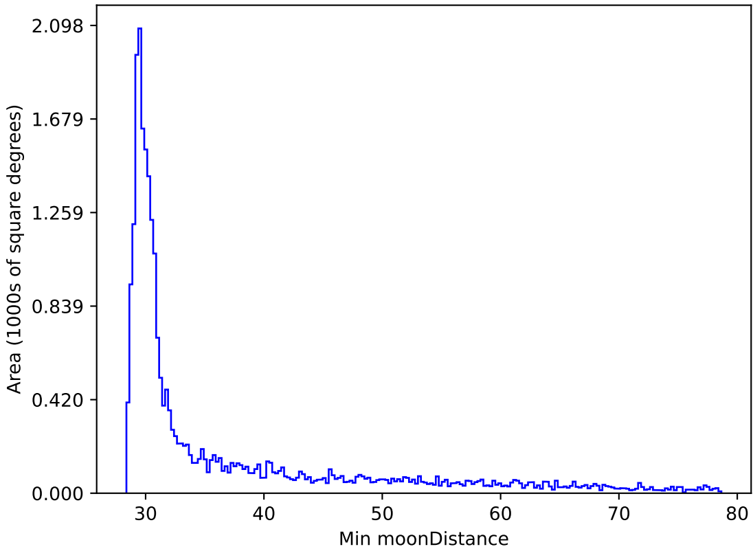
extra_ss_neo3_v3.4_10yrs All sky z band: Min moonDistance
