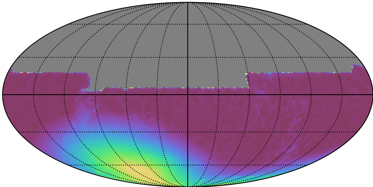
extra_ss_neo3_v3.4_10yrs All sky y band: Min moonDistance
