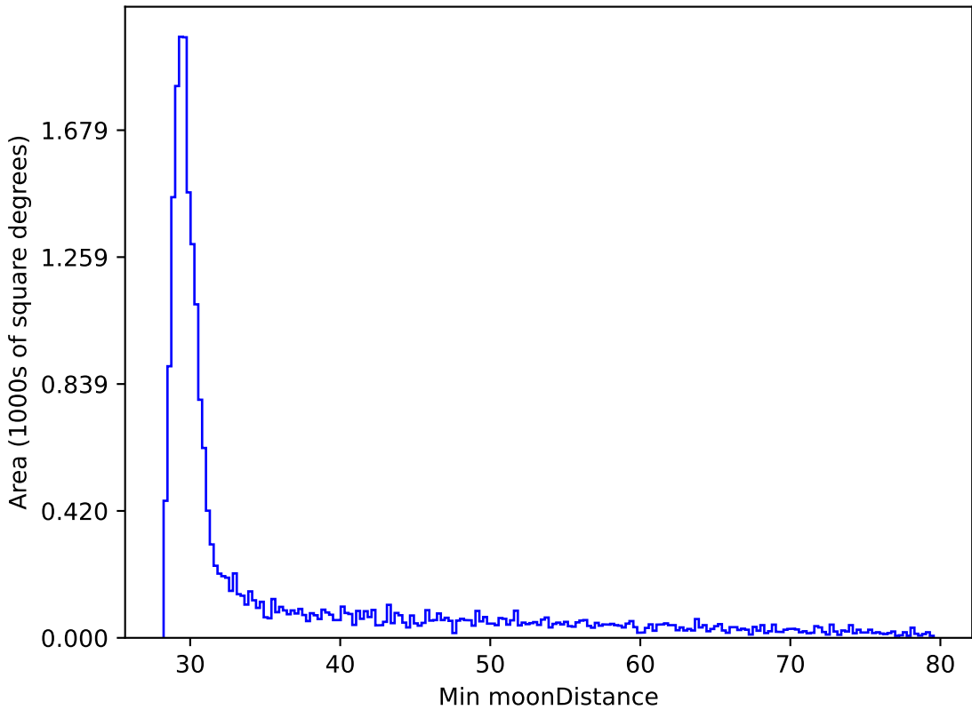
extra_ss_neo3_v3.4_10yrs All sky y band: Min moonDistance
