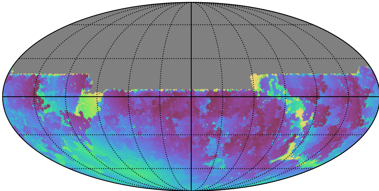
extra_ss_neo3_v3.4_10yrs All sky u band: Min moonDistance
