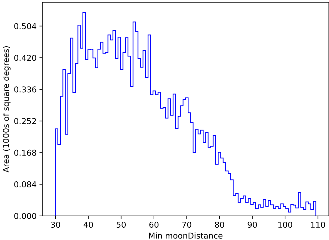
extra_ss_neo3_v3.4_10yrs All sky u band: Min moonDistance
