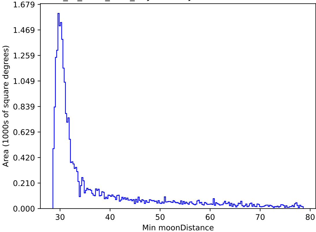
extra_ss_neo3_v3.4_10yrs All sky i band: Min moonDistance
