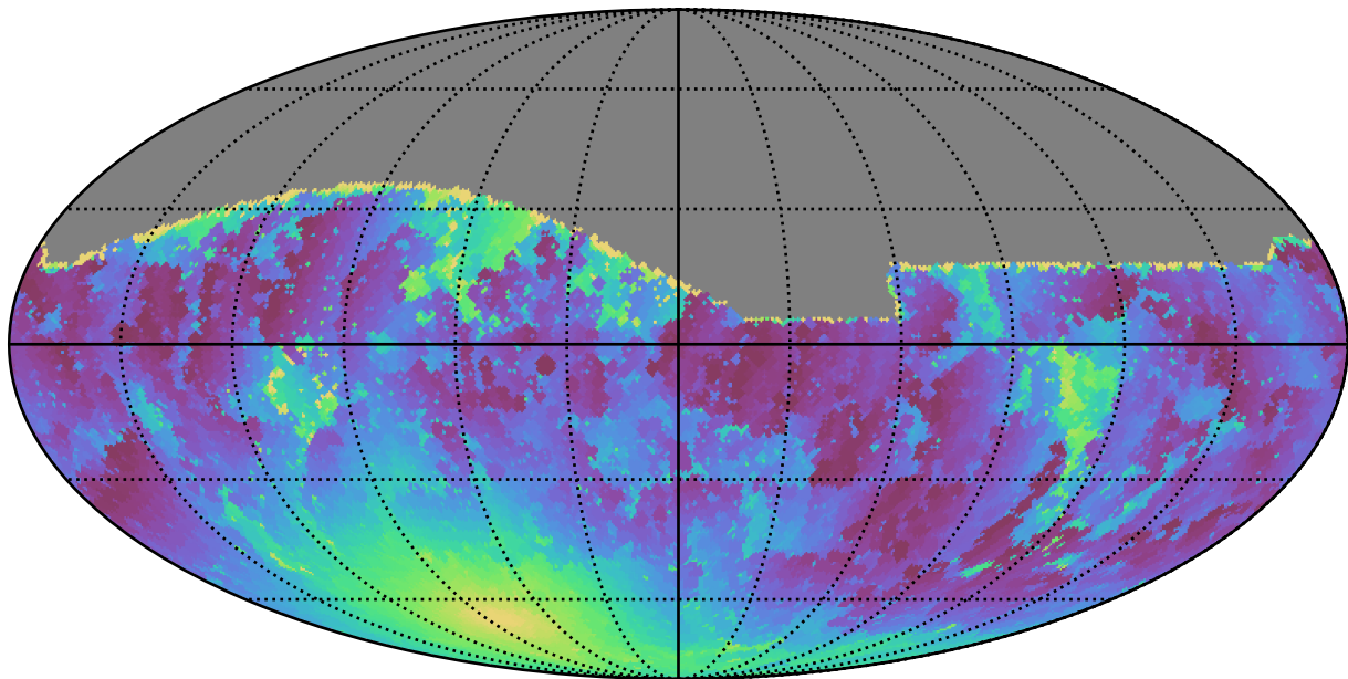
extra_ss_neo3_v3.4_10yrs All sky g band: Min moonDistance
