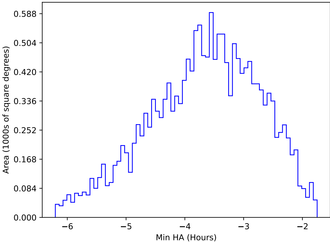
extra_ss_neo3_v3.4_10yrs WFD y band: Min HA
