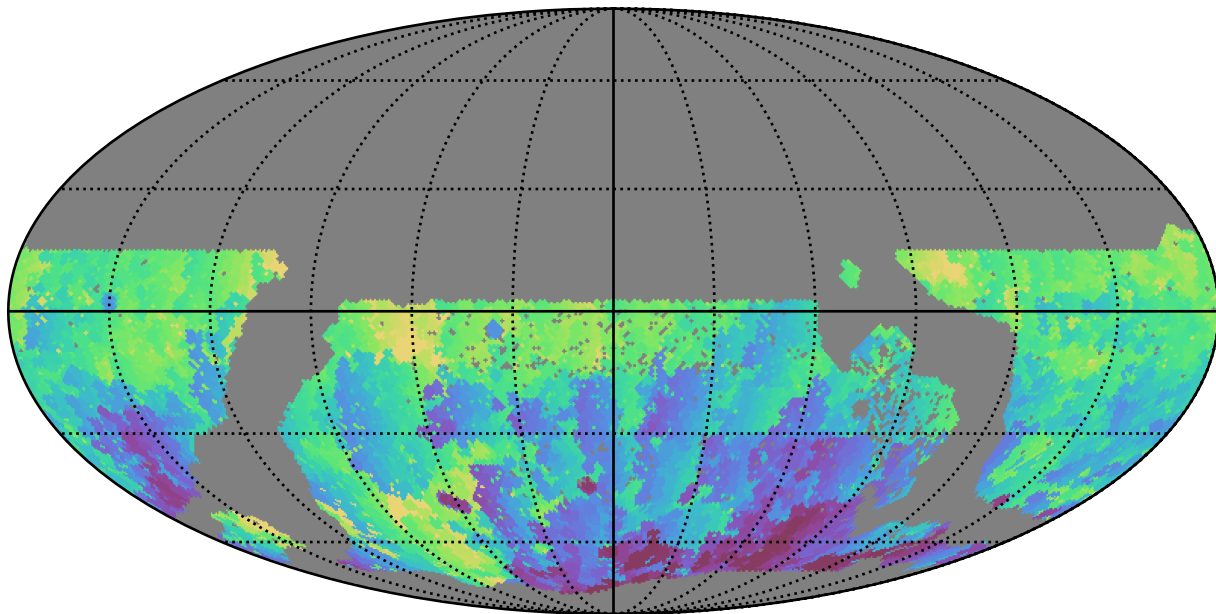
extra_ss_neo3_v3.4_10yrs WFD u band: Min HA
