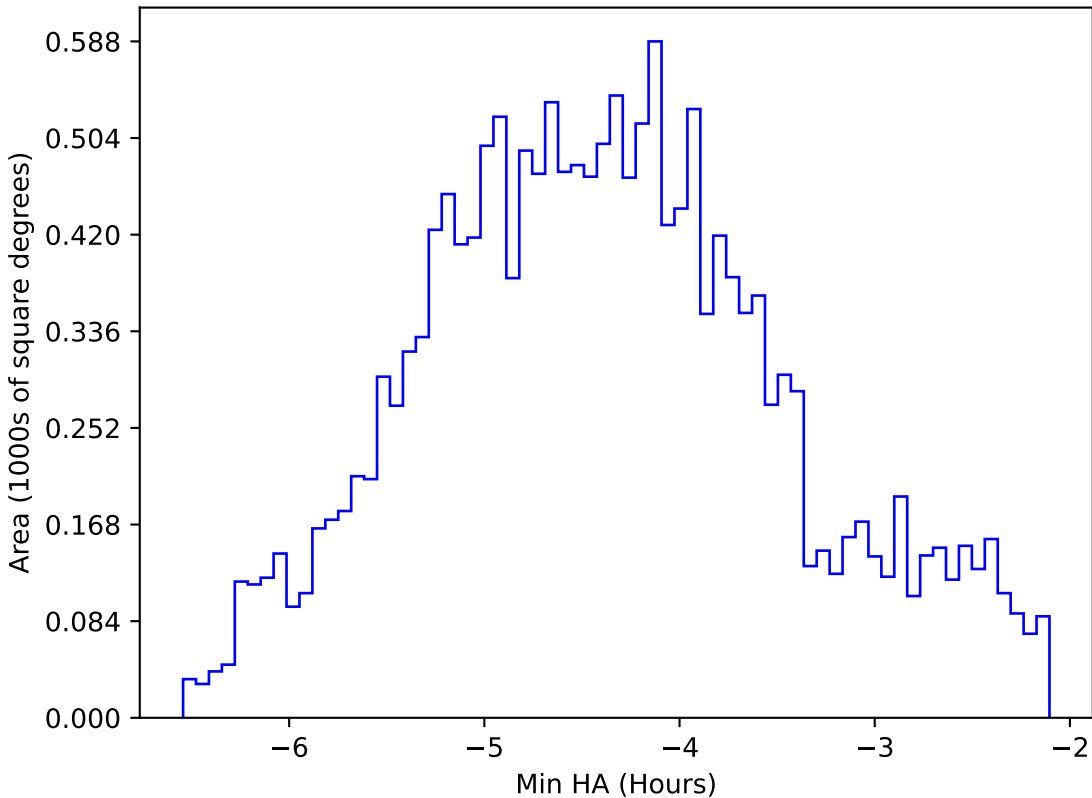
extra_ss_neo3_v3.4_10yrs WFD i band: Min HA
