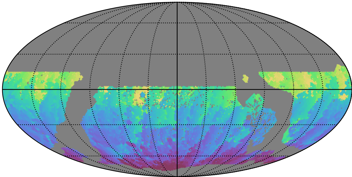
extra_ss_neo3_v3.4_10yrs WFD g band: Min HA
