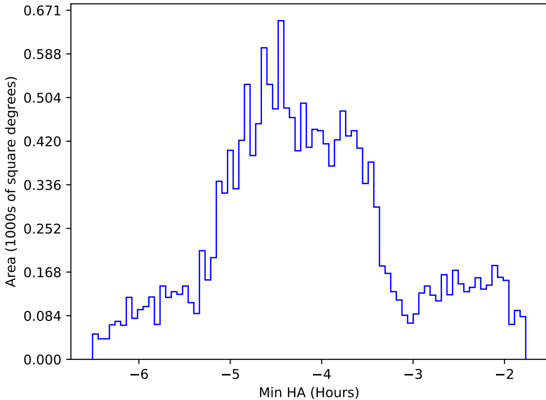
extra_ss_neo3_v3.4_10yrs WFD g band: Min HA
