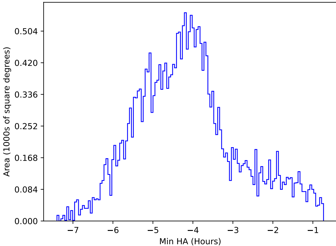
extra_ss_neo3_v3.4_10yrs All sky z band: Min HA
