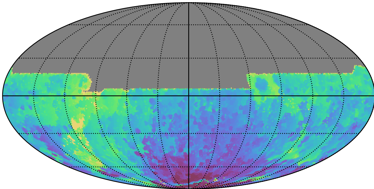
extra_ss_neo3_v3.4_10yrs All sky y band: Min HA
