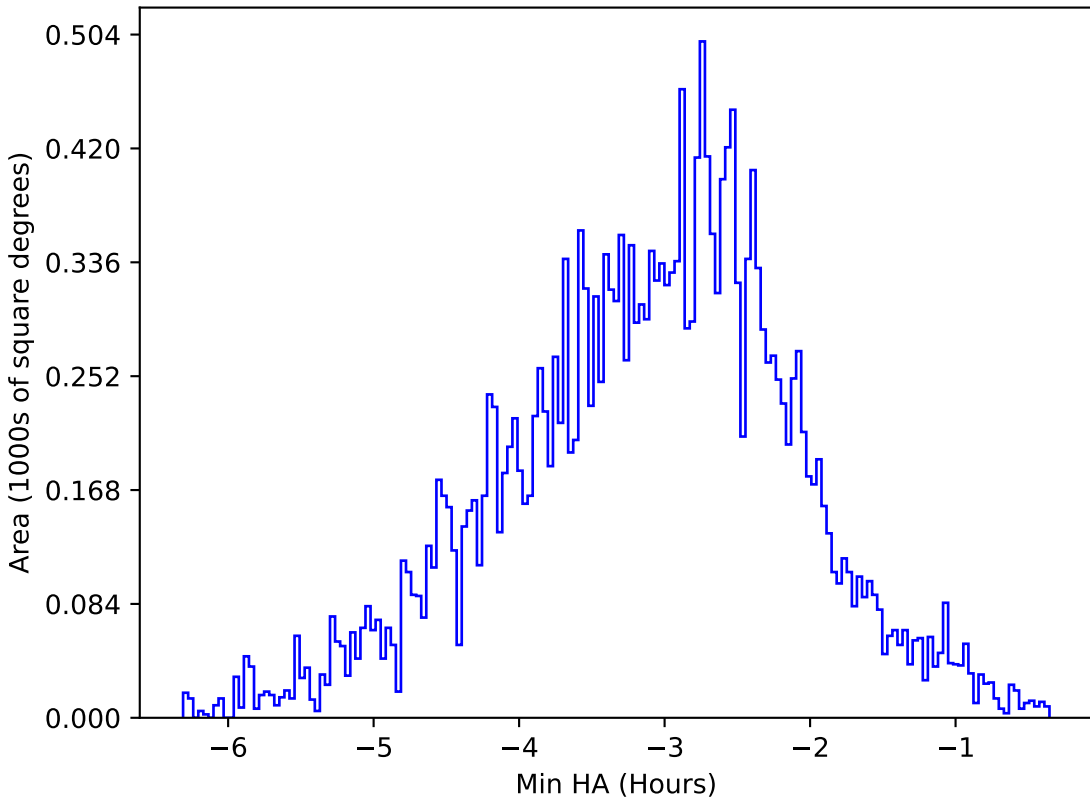
extra_ss_neo3_v3.4_10yrs All sky u band: Min HA
