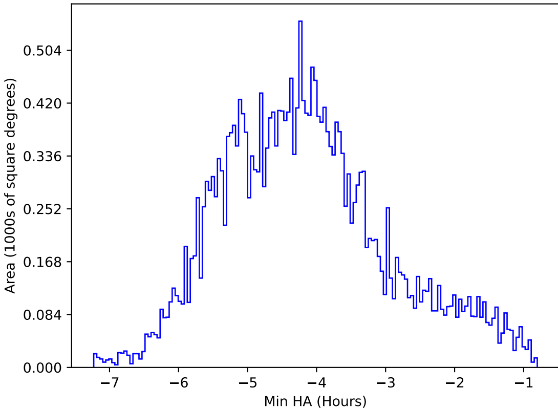
extra_ss_neo3_v3.4_10yrs All sky r band: Min HA
